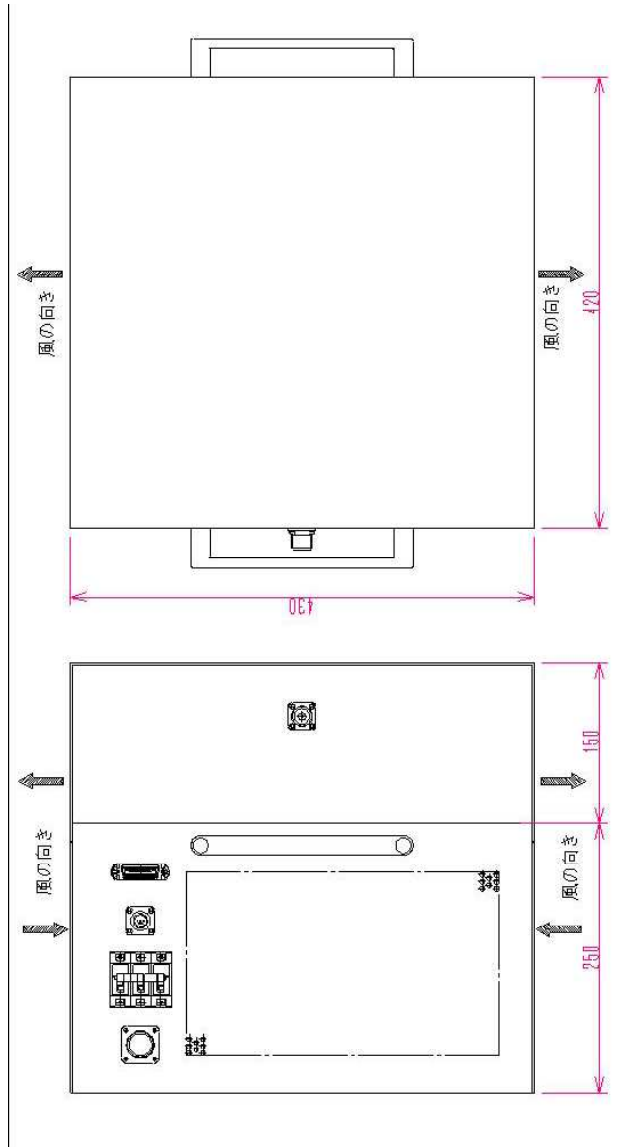
参考外形図
